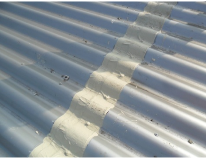
De plaatnaden voorzien van het scheuverbruggende en waterdichte membraan
